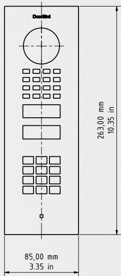
Frontblende
