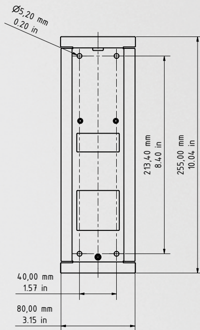
Unterputzgehäuse
