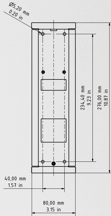
Unterputzgehäuse
